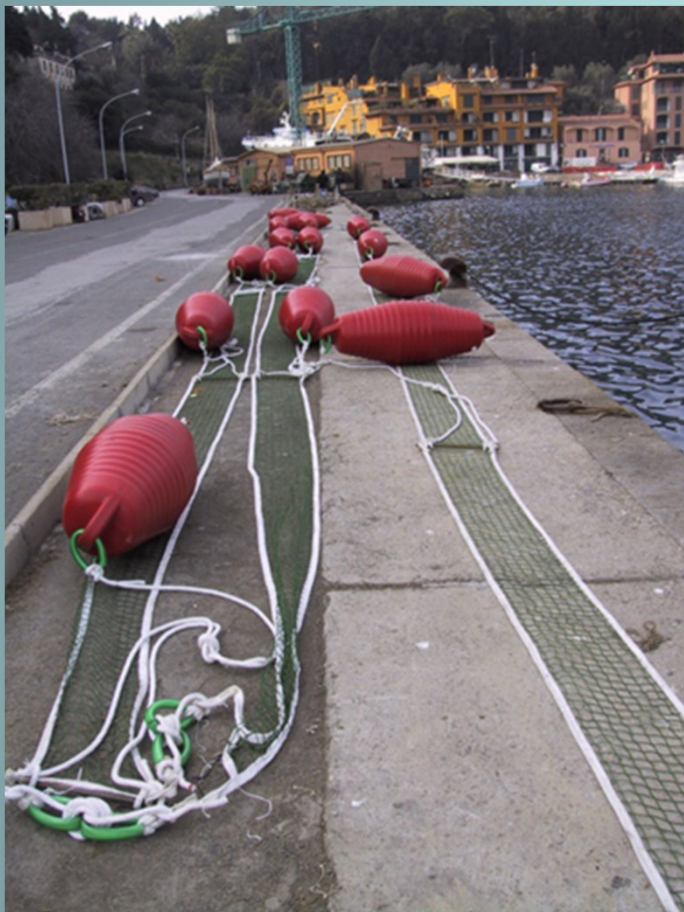
Pannelli in rete pronti per essere installati sui long line
